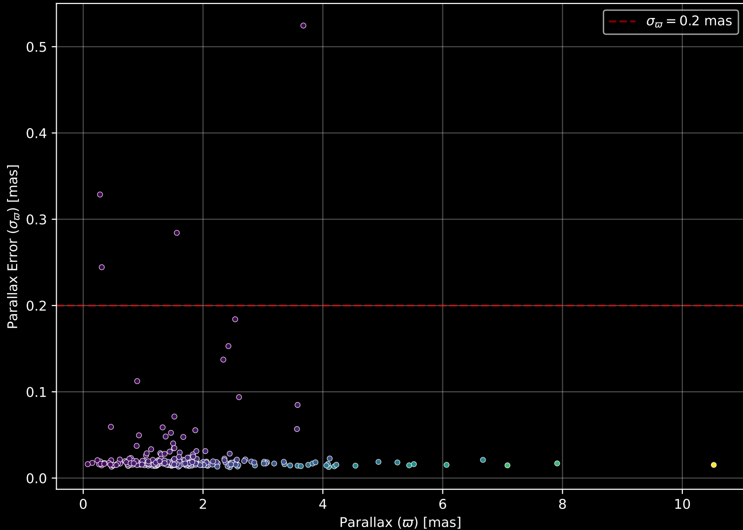
GALAH DR4 Field: [1013] Parallax Quality (n= 285)
