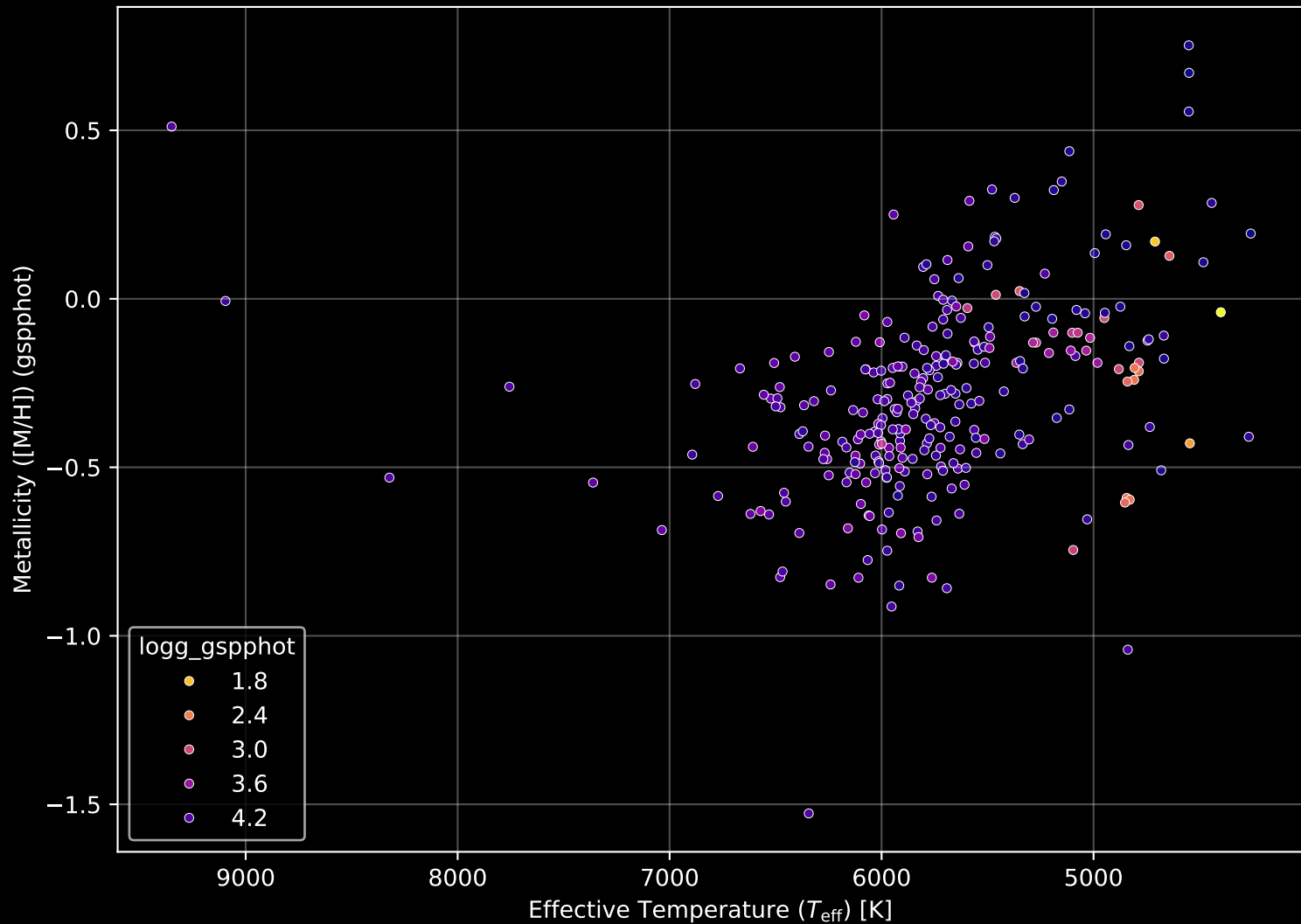
GALAH DR4 Field: [1013] Stellar Population Parameters (n= 285)
