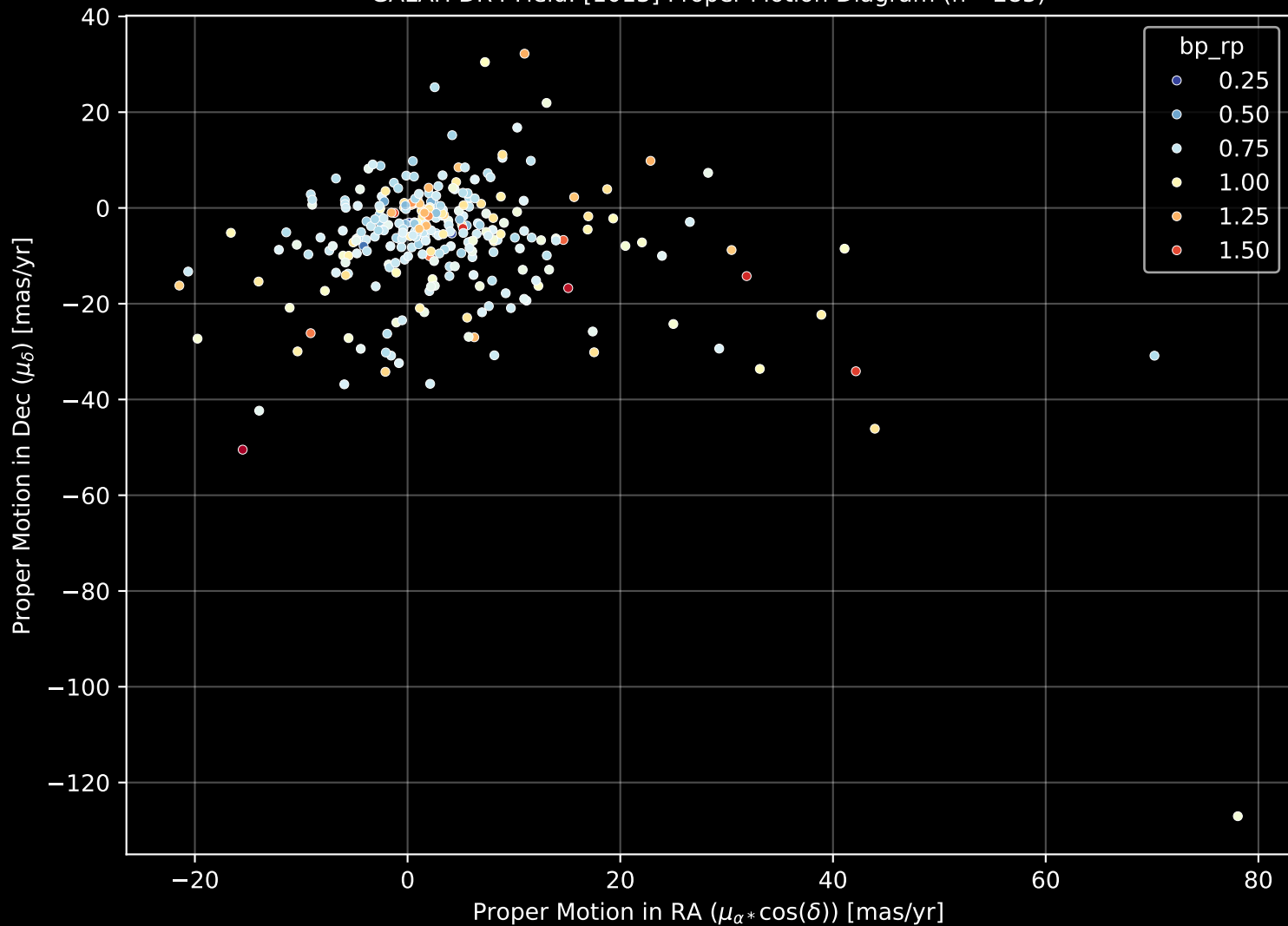
GALAH DR4 Field: [1013] Proper Motion Diagram (n= 285)
