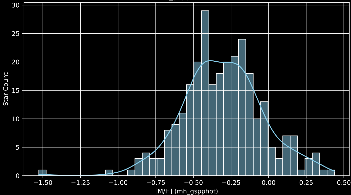
GALAH DR4 Field: [1013] [M/H] (mh_gspphot) (n= 281)
